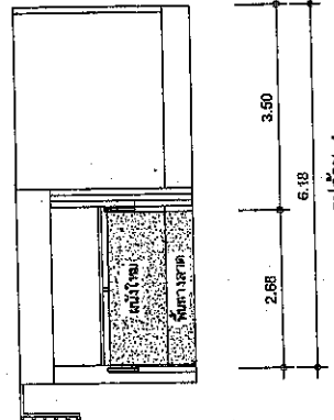
รูปด้าน 4 ขนาดย่อ 1:100
